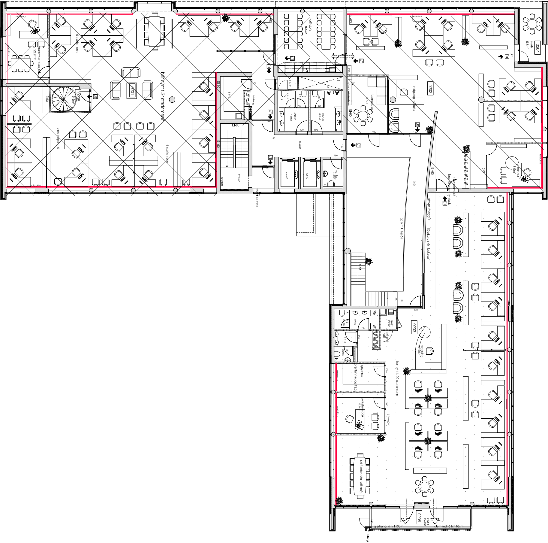
grunnmynd 2. hæð, möguleg skiping og nýting
